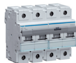
INTERRUPTOR AUTOMÁTICO MAGNETOTÉRMICO SERIE HM
