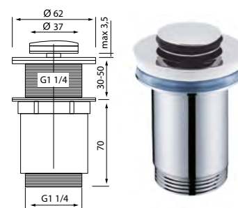
VÁLVULA "CLICK-CLACK" MINI
