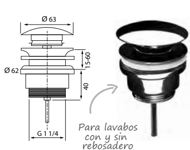
VÁLVULA "CLICK-CLACK" (LAVABO-BIDÉ)
