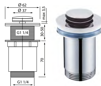
VÁLVULA "CLICK-CLACK" MINI
