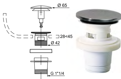
VÁLVULA "CLICK-CLACK" PARA LAVABO Y BIDÉ
