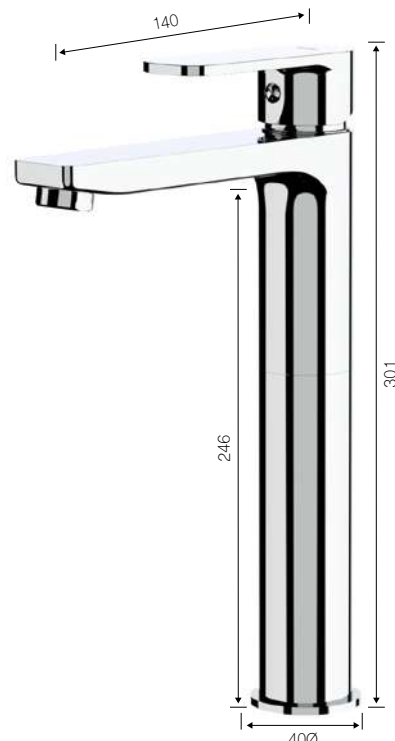
MONOMANDO LAVABO ALTO CABEL PRO CROMO
